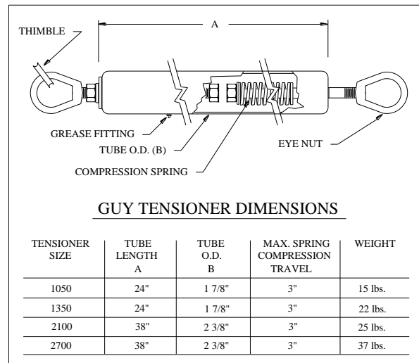
Fig. A-9. Guy Tensioner
